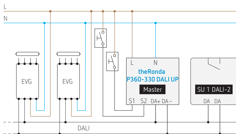
Intégration d'un relais externe DALI
