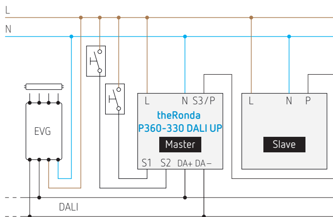
Montage en parallèle maître-esclave
