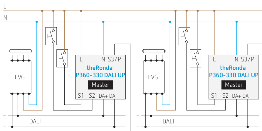
Montage en parallèle maître-maître
