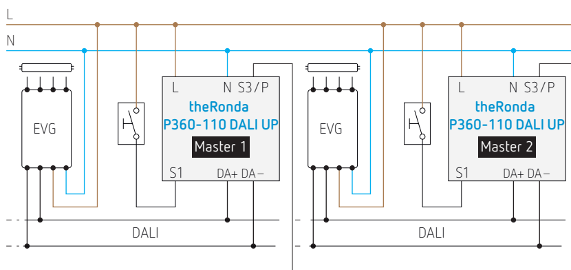
Montage en parallèle maître-maître
