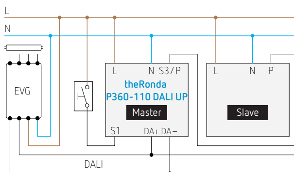
Montage en parallèle maître-esclave
