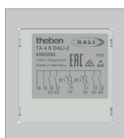
TA4 S DALI-2, 4-voudige DALI-2 toetsinterface UP
