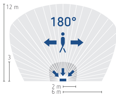
theLeda B dual sensor BK, bewegingsdetectiemodule te bevestigen op de ledstraler (optioneel)
