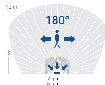
theLeda B dual sensor BK, bewegingsdetectiemodule, te bevestigen op de ledstraler theLeda B dual
