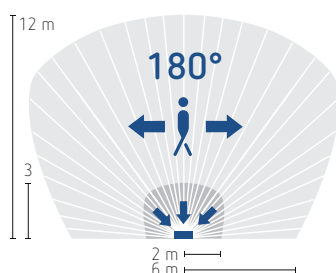
theLeda B dual sensor BK, module de détection de mouvement, à fixer sur le projecteur led (en option)
