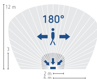
theLeda B dual sensor WH, bewegingsdetectiemodule, te bevestigen op de ledstraler theLeda B dual
