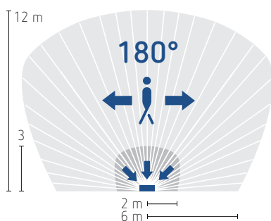
theLeda B dual sensor BK, bewegingsdetectiemodule, te bevestigen op de ledstraler theLeda B dual (optioneel)
