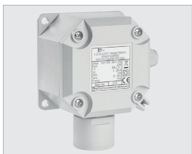
Sensor 4 tot 20 mA voor toepassing zonder ATEX-classificatie
