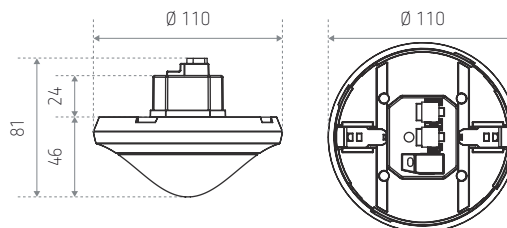
FRAME 110A WH 9070912, boîtier pour montage apparent
