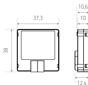
907.0.489, temperatuursensor in behuizing met scharnierend deksel voor het meten van de temperatuur op pijpen en gebogen oppervlakken
