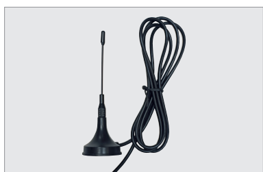
ANT 868 , antenne RF 433 MHz pour T6S en option, intérieur et extérieur; connecteur SMA-mâle avec câble de 90 cm RG-174/50 Ω, gain: 2,5 dBi (max. 50 W); base magnétique, dimension: Ø 13 × 172 mm
