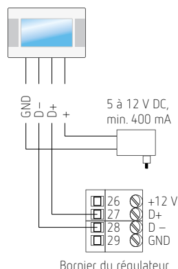
Bornier du régulateur
