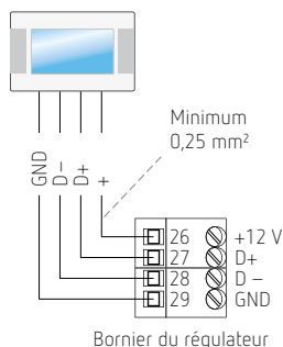
Bornier du régulateur
