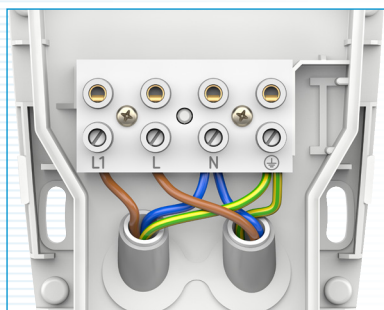
Socle spacieux
