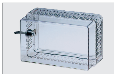
473.051.000.006 (SGH 473), capot à serrure 194 × 120 × 85 mm. Option: 2 clés, réf. 007.57.0730.000
