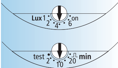
PresenceLight 360 , plafondmontage
