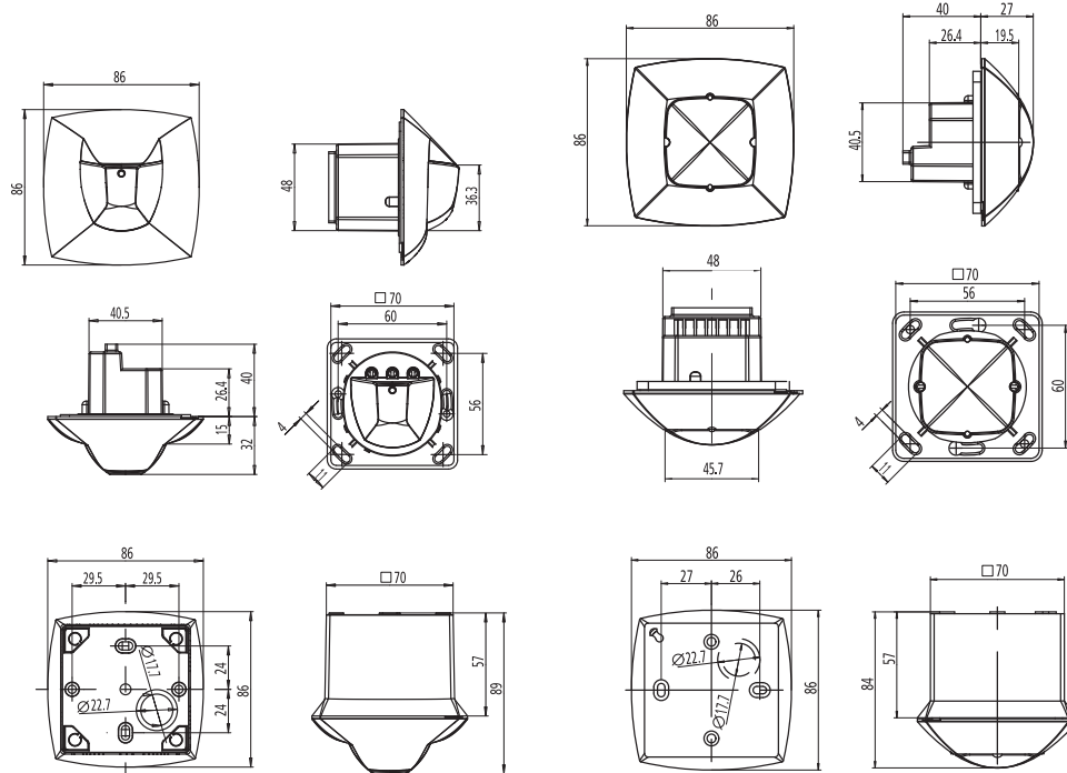
Montage op opbouwframe 907 0 513, in optie PresenceLight 180
