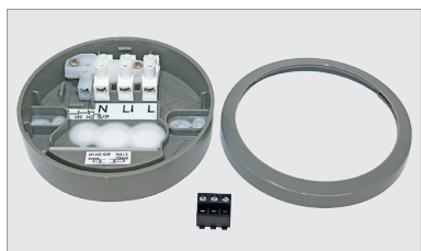
Surface box LUXA 103 GR, grijs opbouwframe in optie
