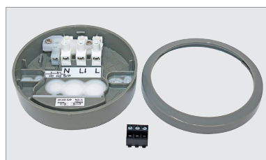
Surface box LUXA 103 GR, cadre gris pour montage apparent
