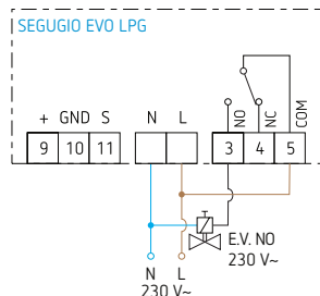
Avec électrovanne normalement ouverte à réarmement manuel 230 V
