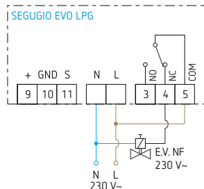
Avec électrovanne normalement fermée à réarmement manuel 230 V
