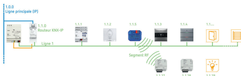
Le coupleur de médias relie les composants câblés aux composants radio (RF). Le firmware actuel du coupleur de médias prend en charge la segmentation des lignes dans ETS 6 et permet ainsi d'équiper facilement les systèmes existants de composants RF.
