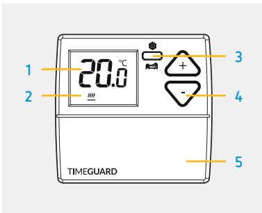
TRT047N: thermostaat zender en ontvanger vooraf afgestemd
