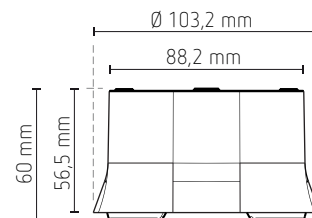
Behuizing voor opbouwmontage 907 0 912 - 110A WH
